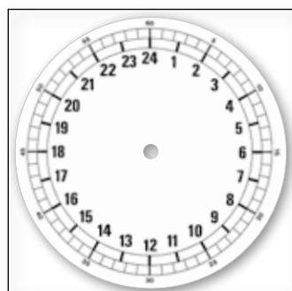
24-uurs wijzerplaat Wit gelakt aluminium met opgedrukte cijfers. Buiten-Ø 185 mm, midden-gat-Ø 10,5 mm. 1 mm dik. Voor wijzerlengte 72-80 mm. 335012 26,90
