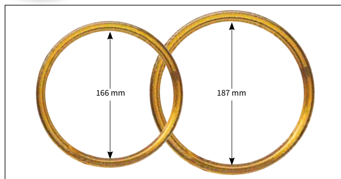
Losse afsluitranden Voor reguleur wijzerplaten. Gepolijst messing. Buiten-Ø Binnen-Ø Buitenhoogte Binnenhoogte Wijzerpl. Ø Bestelnr. Prijs 182 mm 166 mm 15 mm 8 mm 180 mm 334978 47,90 205 mm 187 mm 16,5 mm 10 mm 204 mm 334979 54,90
