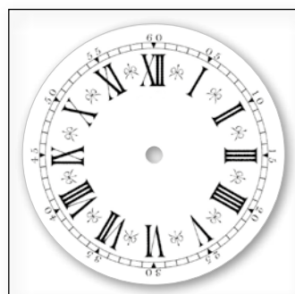
Wijzerplaat Wit gelakt aluminium met opgedrukte zwarte cijfers. Buiten-Ø 178 mm, 0,6 mm dik, plat. Middengat-Ø 10,2 mm. Voor wijzerlengte 65-80 mm. 334966 10,90
