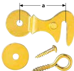
Türhaken vermessingt, für große Wand- und Standuhren. Einschl. Ring- und Rundkopfschraube sowie U-Scheibe. Maß a = 25 mm. 2 Stück/Pckg. 222287 4,40
